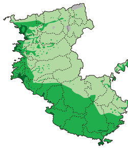
南海トラフ巨大地震
