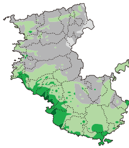
東海・東南海・南海3連動地震
