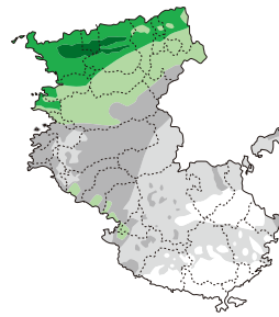
中央構造線による地震
