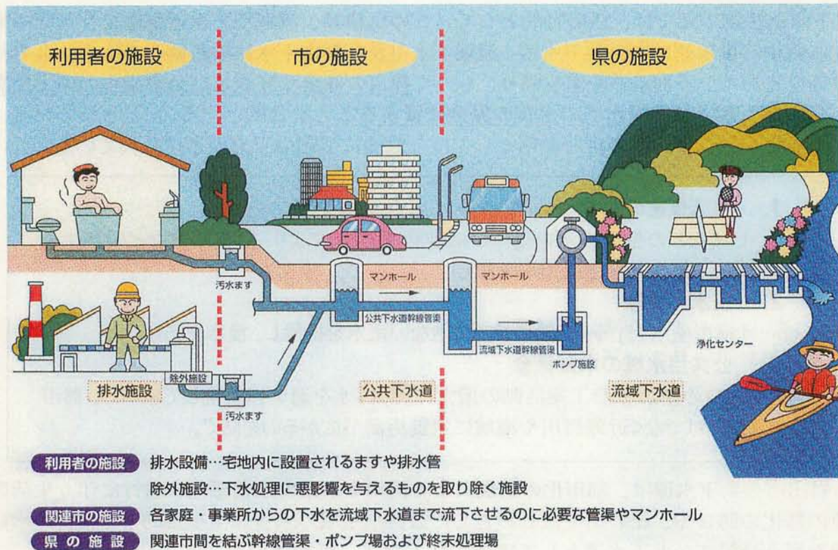
図4-1 下水道のしくみ（流域下水道）
