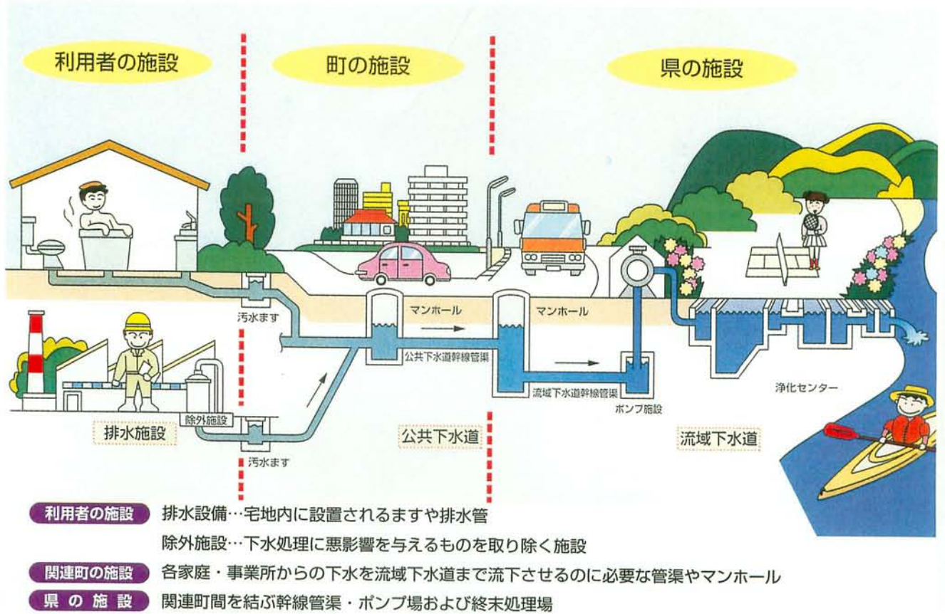
図2-1 下水道のしくみ（流域下水道）
