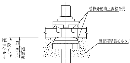
高さ調整部詳細図 S=1:2
