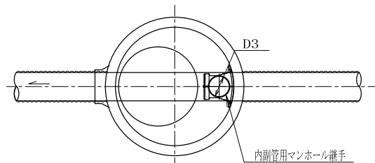
副管寸法（硬質塩化ビニール管）
