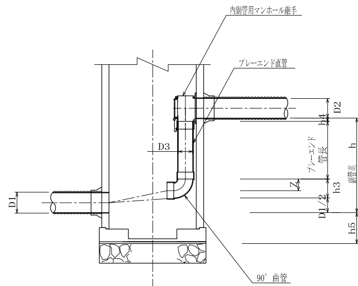
断面図
