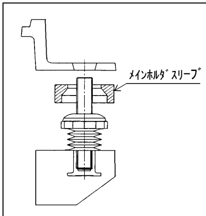
④メインホルダスリーブ取付け
