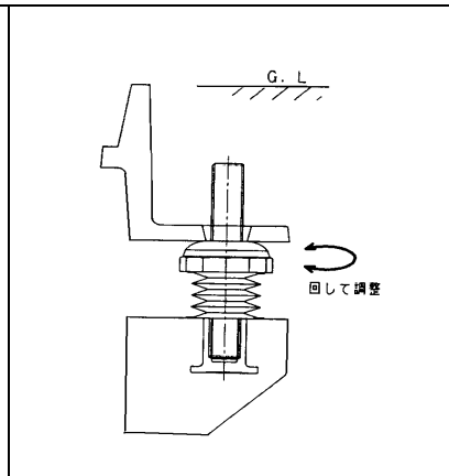
③受枠高さ調整
