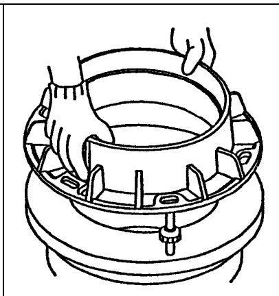
④メインホルダスリーブ取付け
